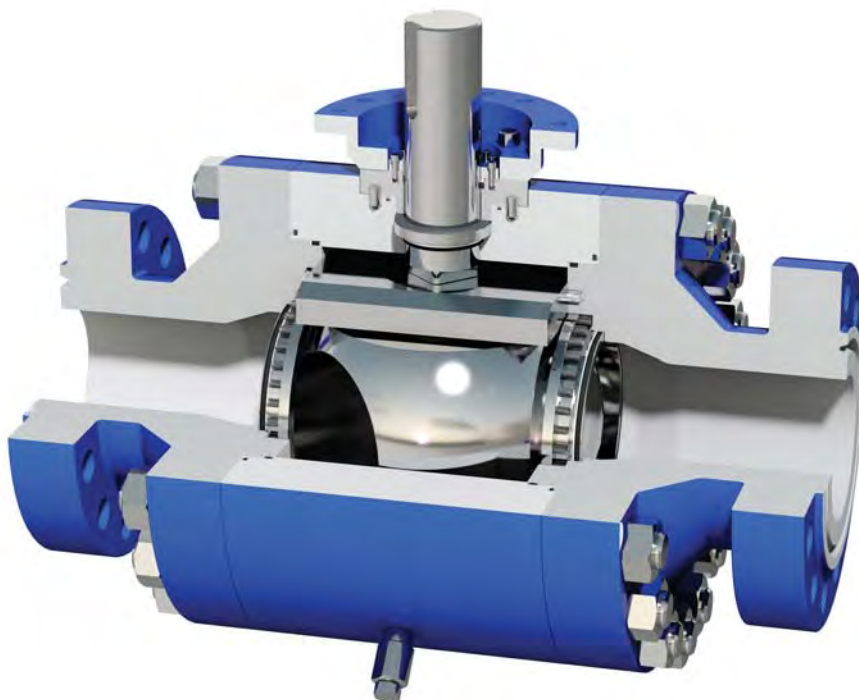
Alle Kugelhähne von Hartmann Valves verfügen über ein rein metallisches Dichtsystem.
